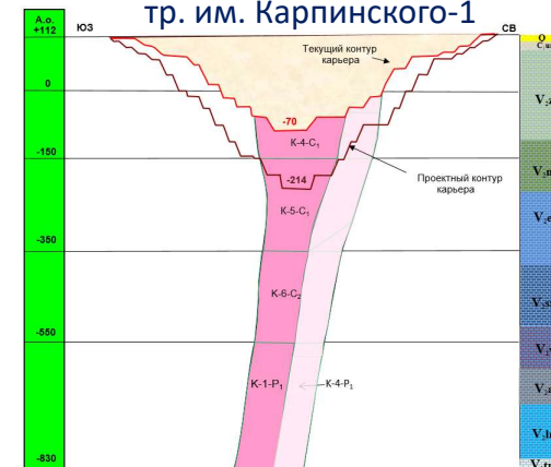
Положение горных работ на тр. им. Карпинского-1
