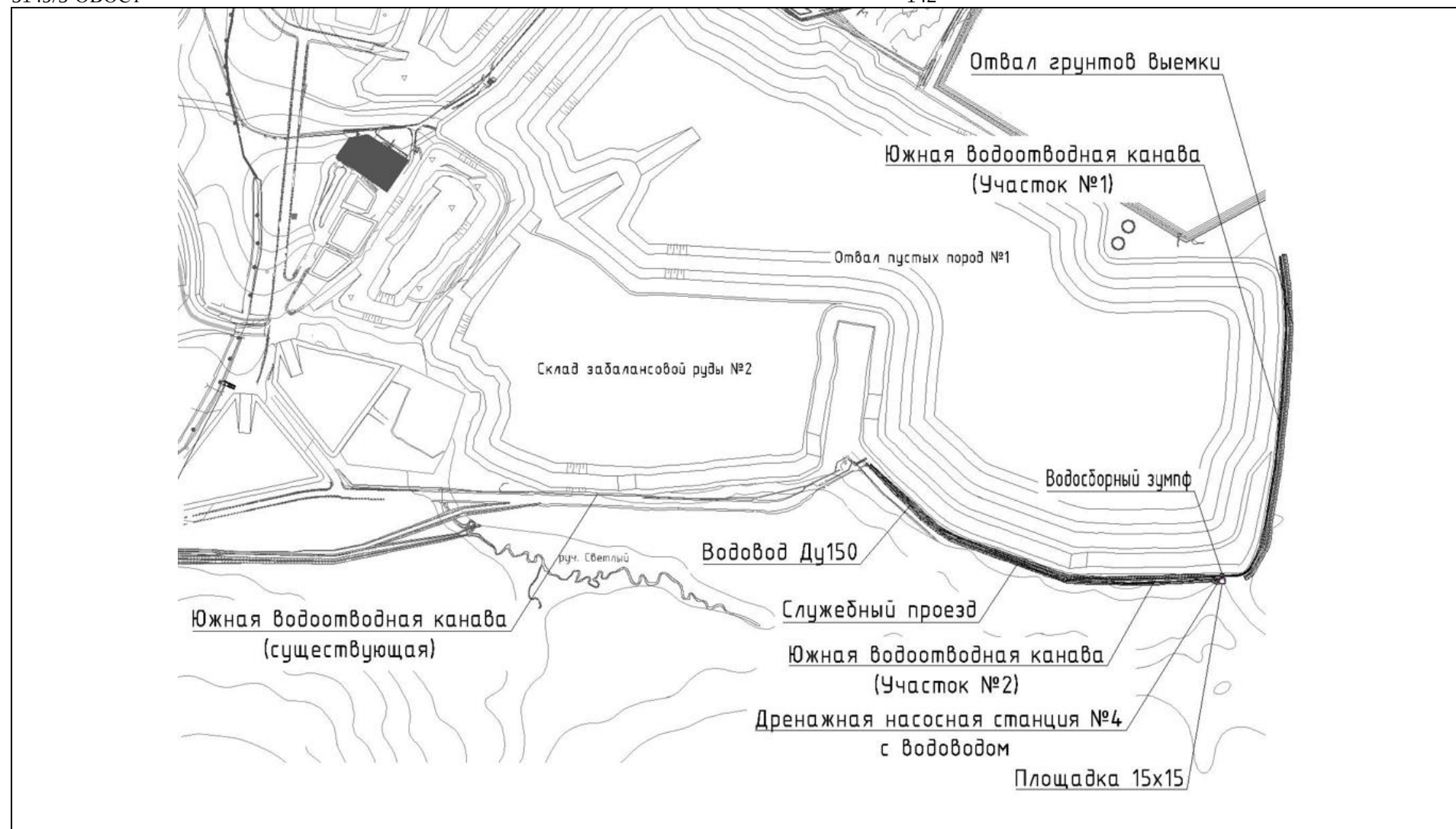
Рисунок 3.2 – Схема расположения проектируемых водоотводных сооружений (отвала пустых пород №1)
