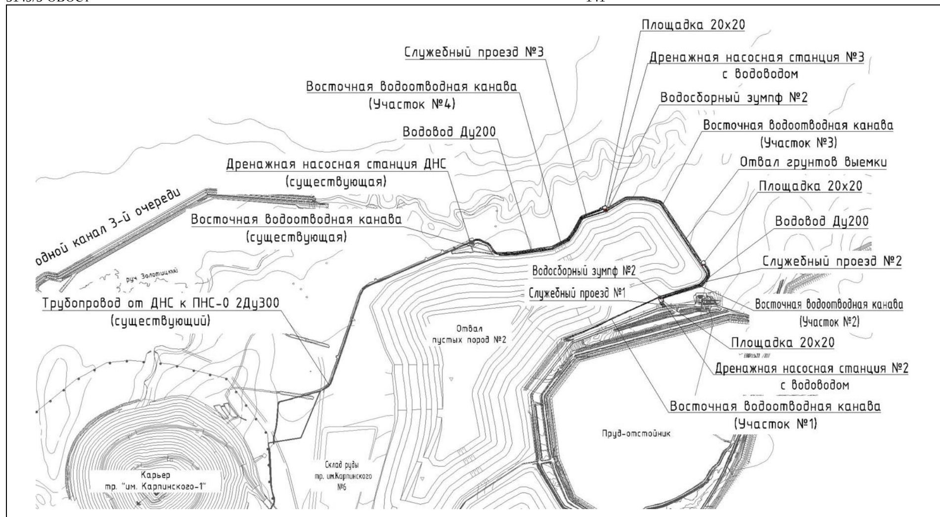
Рисунок 3.1 – Схема расположения проектируемых водоотводных сооружений (отвала пустых пород №2)
